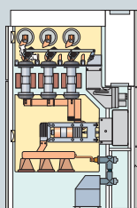
Ячейка силового выключателя IK ESS
