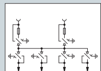
Схема 62
