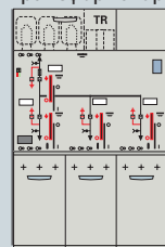
Схема 71
