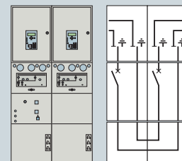
Секционные ячейки DSS
