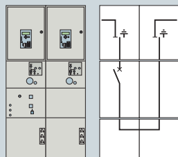
Ячейка разъединителя Секционные ячейки ESS
