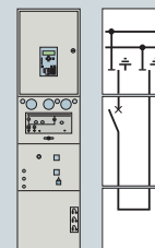
Ячейка с шиносоед. выключателем DSS
