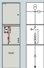
Ячейка выключателя нагрузки
