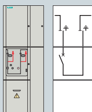
Секционная ячейка ESS
