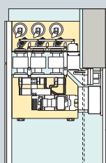
Секционная ячейка ESS
