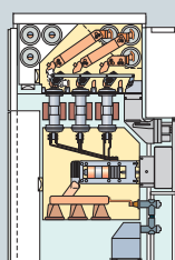
Ячейка силового выключателя IK DSS
