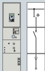
Ячейка силового выключателя ESS
