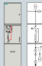
Ячейка контактора
