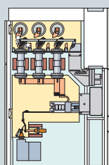
Ячейка силового выключателя AK ESS
