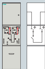
Секционная ячейка
