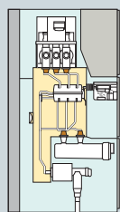
Ячейка выключателя нагрузки
