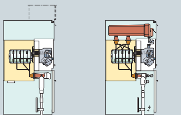
Фидер кольцевого кабеля
