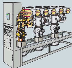
Ячейка силового выключателя DSS
