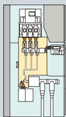
Ячейка разъединителя
