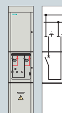
Ячейка с шиносоед. выключателем DSS
