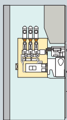
Секционная ячейка
