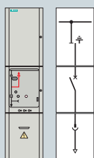
Ячейка силового выключателя AK ESS
