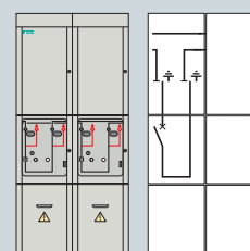
Секционные ячейки DSS
