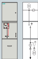
Ячейка разъединителя
