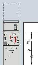
Ячейка силового выключателя Тип LST1
