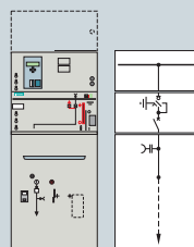
Ячейка силового выключателя LS11 с ЗАН6
