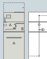
Измерительная ячейка ME1
