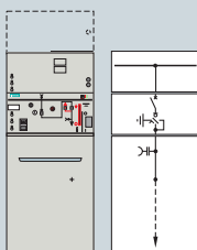
Ячейка силового выключателя LS1 с ЗАН5
