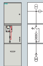
Измерительная ячейка
