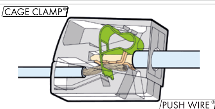
Сторона монтажа: вставьте зачищенный однопроводный проводник в круглое отверстие до упора.
