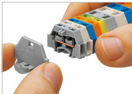
Установка торцевой пластины.
