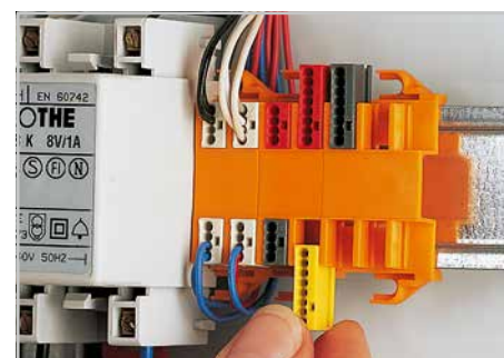
Вставка клеммы в монтажный адаптер.
