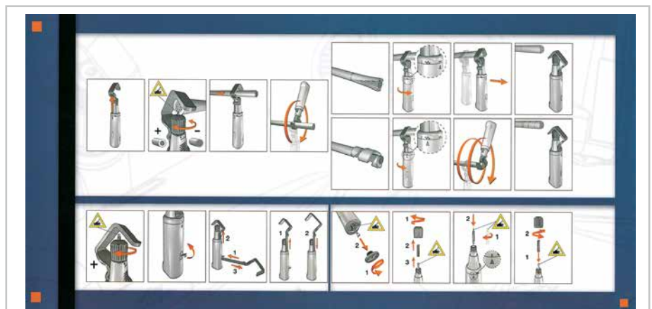
Инструкция для инструмента для зачистки изоляции 206-174
