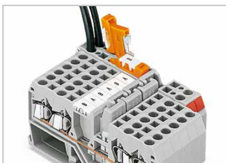
Ступенчатые перемычки для сложных схемотехнических решений – нажимайте на перемычки до их полной установки.
