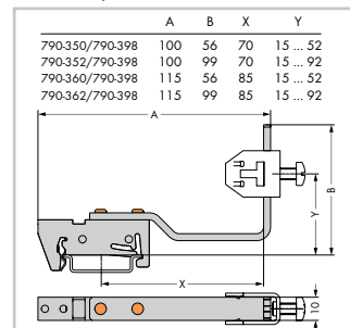
Обзор: размеры гибких держателей шин
