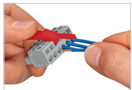
Монтаж проводников перпендикулярно действию зажима CAGE CLAMP®
