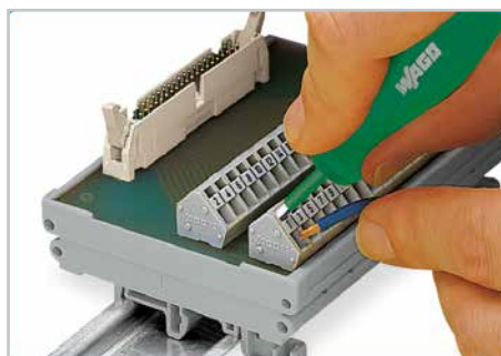
Подсоединение проводника методом фронтального монтажа
