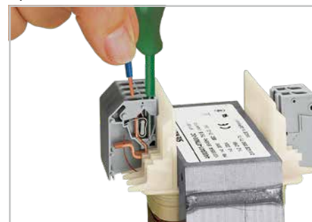
Присоединение проводников (сторона вторичной обмотки)
