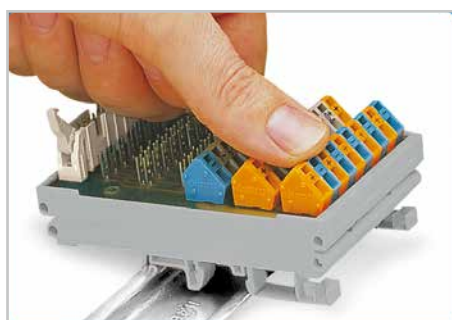
Закрепление модуля на DIN-рейке.
