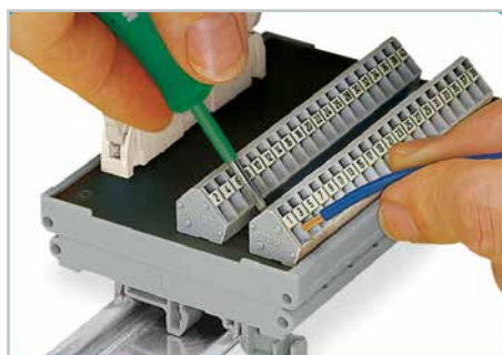
Подсоединение проводника - «боковой монтаж»
