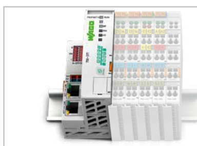
Конструкция корпуса без питания системы
