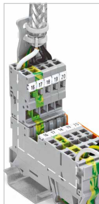
Зажим экрана
