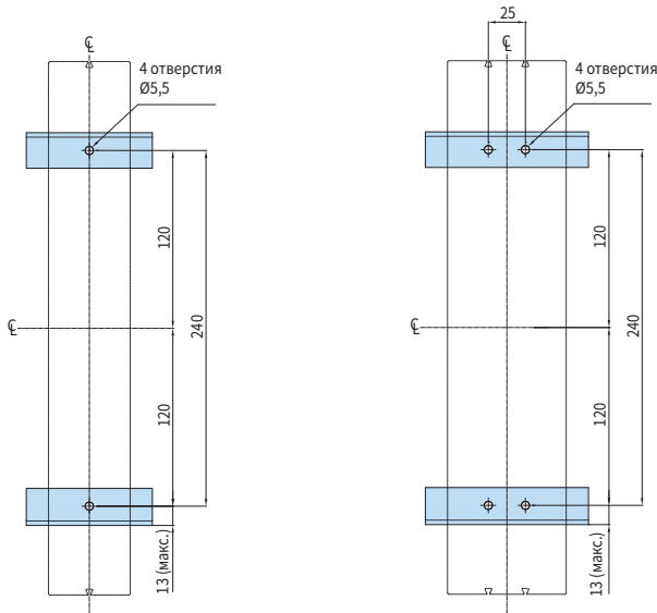
Монтажный чертеж
