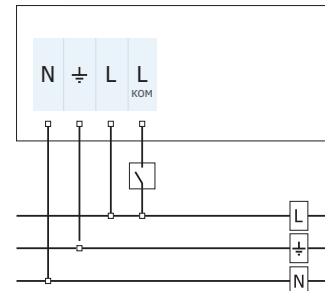
Схема включения светильника с блоком аварийного питания.
