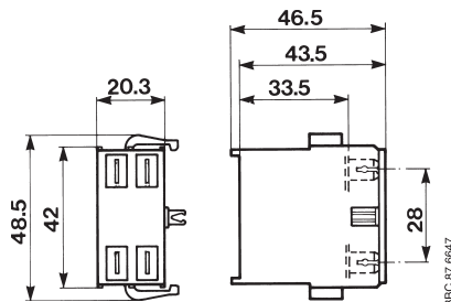
Блок вспомогательных CA 6- F со штырьковыми соединениями
