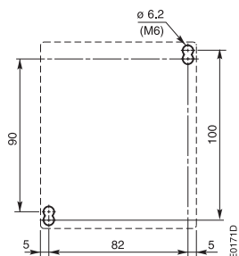
Установочные размеры для A 45, A 50, A 75, AF 45, AF 50, AF 75
