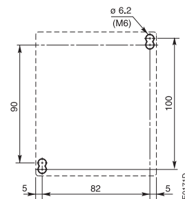
Установочные размеры для АЕ 45, АЕ 50, АЕ 75, ТАЕ 45, ТАЕ 50, ТАЕ 75
