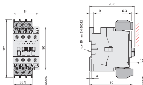
Контакты А 26, (Т) АЕ 26, UA 26 + 2 x LD 26
