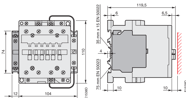
АЕ 45, АЕ 50, АЕ 75, ТАЕ 45, ТАЕ 50, ТАЕ 75 + 2-полюсный блок вспомогательных контактов боковой установки СА1 5
