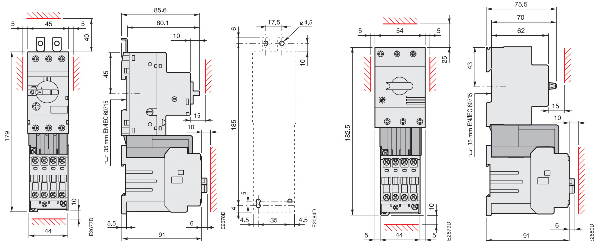
Контакторы AL 9, AL 12, AL 16 + BEA 16/116AL + MS 116
