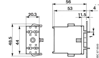
CA 6 + LB 6- CA В 6, В 7 + Тепловое реле Т 7 DU
