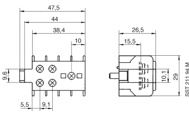
с винтовыми зажимами
