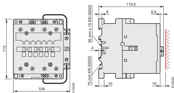
АЕ 45, АЕ 50, АЕ 75, ТАЕ 45, ТАЕ 50, ТАЕ 75
