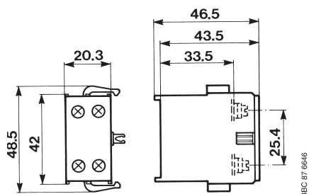
Блок вспомогательных контактов CA 6 с винтовыми зажимами
