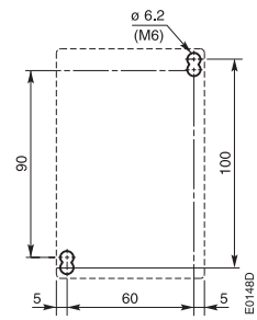
Установочные размеры
