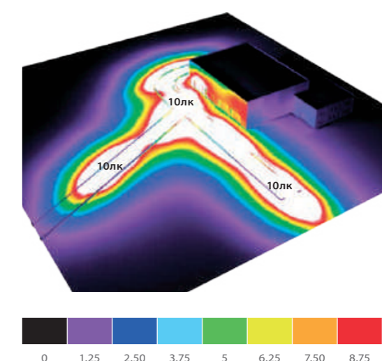
Светодиодные светильники «KEDR 2.0 SKY 75»
