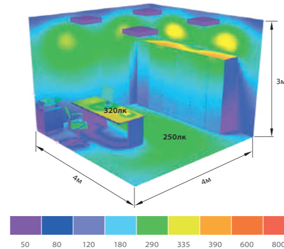
Люминесцентные светильники «ЛВО 4x18»
