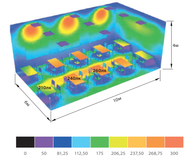
Светодиодные светильники «ОФИС»
