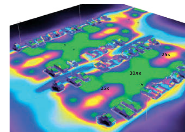
Светодиодные светильники «KEDR 2.0 SKU 100»
