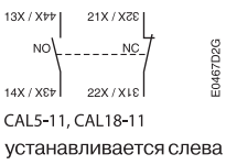
CAL5-11, CAL18-11 устанавливается слева
