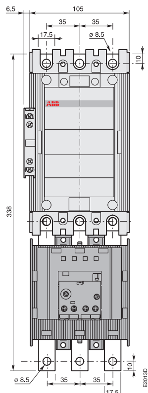
A 145, A 185, AF 145, AF 185 с 1 x CAL 18 + электронное реле перегрузки E 200 DU
