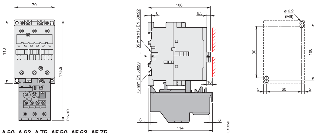
А 50, А 63, А 75, АF 50, АF 63, АF 75 + тепловое реле ТА 75 DU
