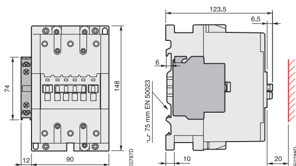
A 95, A 110, AF 95, AF 110 + 2-полюсный блок вспомогательных контактов боковой установки CAL 18
