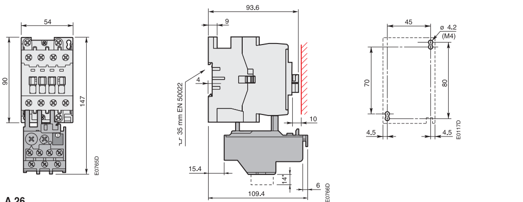
A 26 + тепловое реле TA 25 DU
